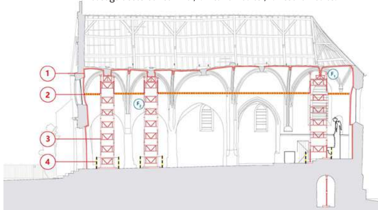
1. Purge éléments instables ; 2. Filets de protection ; 3. Structure d'étalement ; 4. Balisage accès condamné ; I. Inclinomètres ; F. Fissuromètres.
