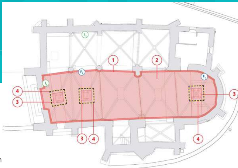
1. Purge éléments instables ; 2. Filets de protection ; 3. Structure d'étalement ; 4. Balisage accès condamné ; I. Inclinomètres ; F. Fissuromètres.
