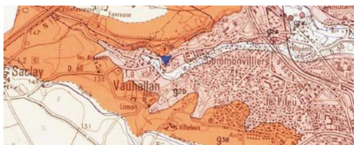
Nature des sols de la zone foncée vers la plus claire : Meulière et Argile à Meulière de Montmorency ; Sable et Grès de Fontainebleau ; Alluvions récentes.
